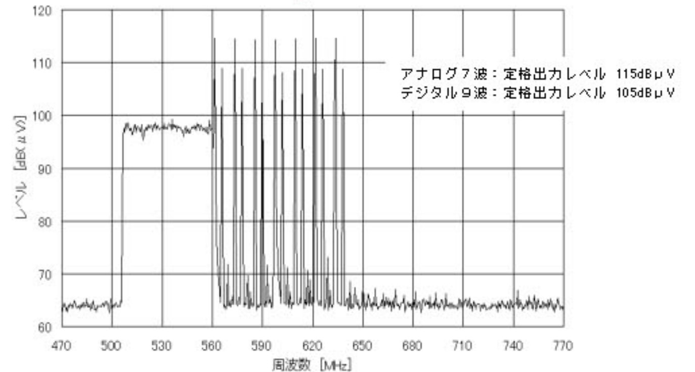
高出力ブースタにアナログ7波+デジタル9波が入った場合
