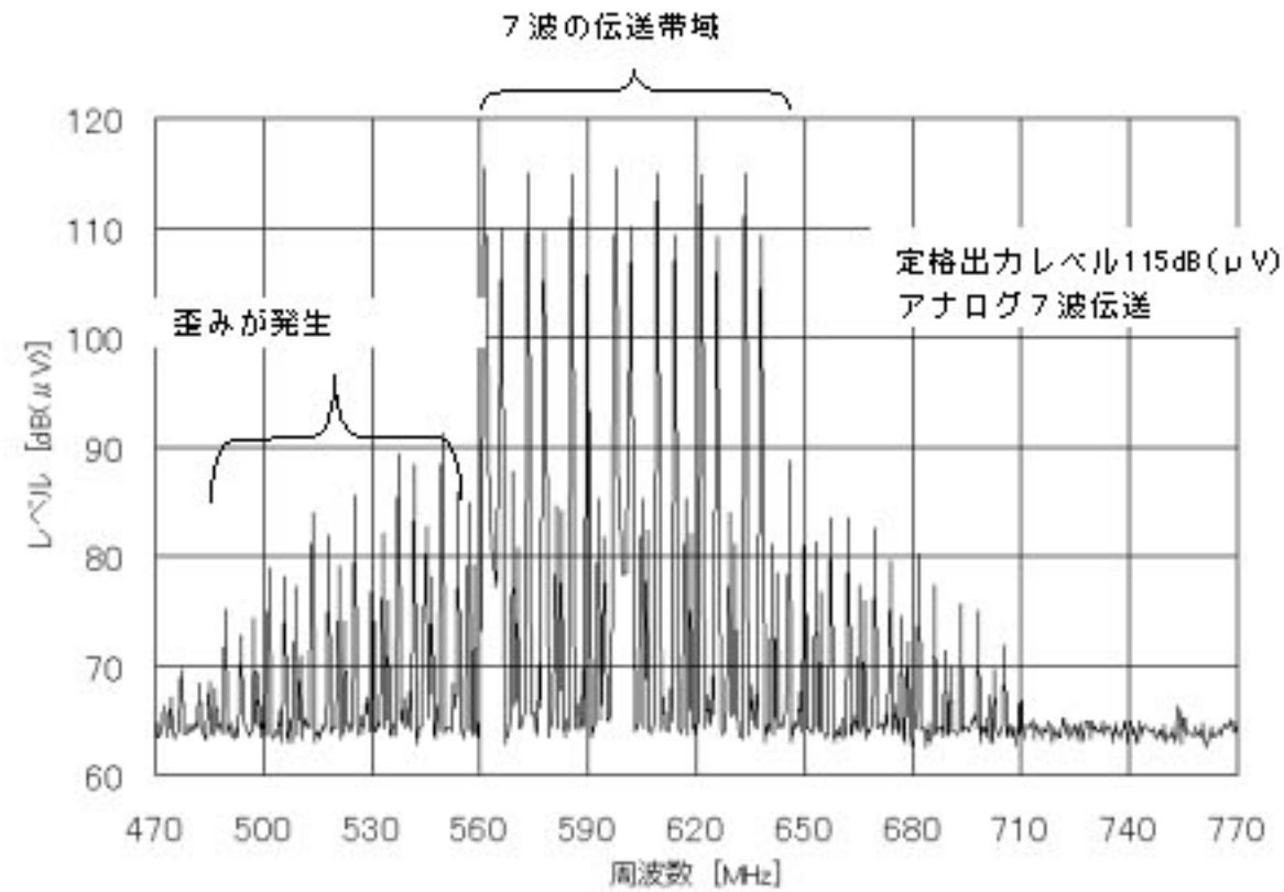
2波伝送仕様の従来ブースタにアナログ7波が入った場合の波形
