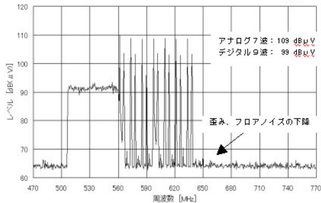
アナログ7波+デジタル9波が入った時に出力レベルを下げた場合
