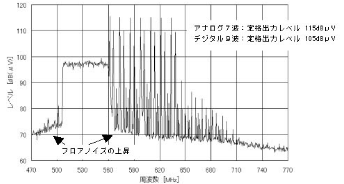
アナログ7波+デジタル9波が入った場合
